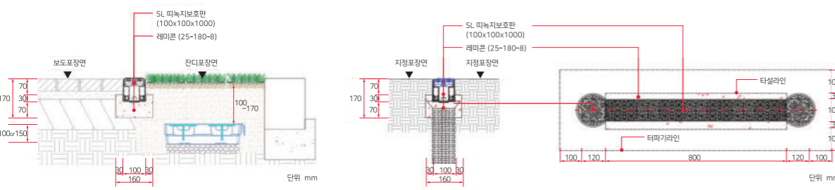
[레미콘 타설 시공 단면도]
