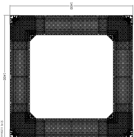
1 가로수보호판 및 보호틀 SCALE : NONE
