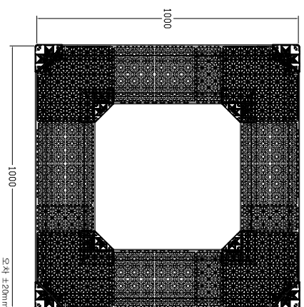
가로수보호판 및 보호틀 SCALE : NONE
