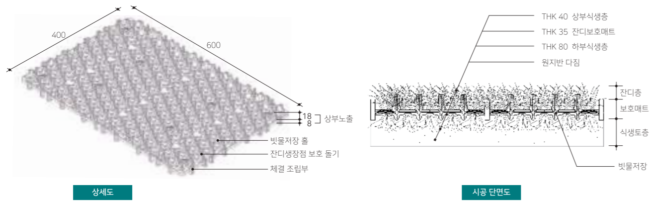
상세도면
