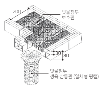
부분 상세도
