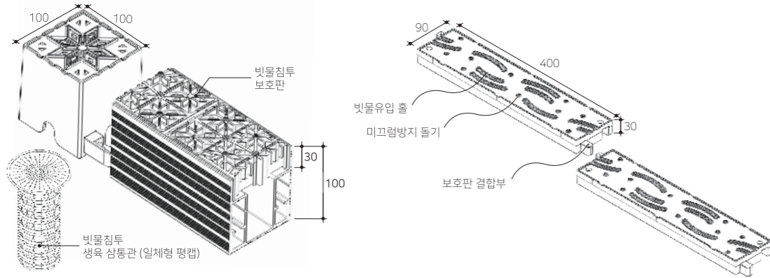
부분 상세도
