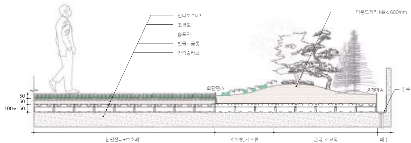
시공 단면도
