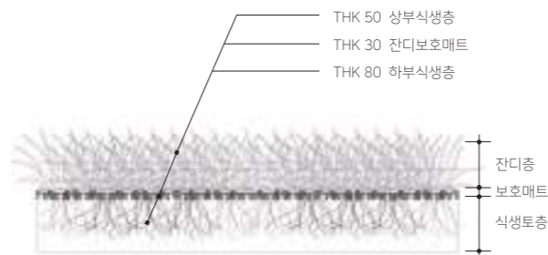
시공 단면도
