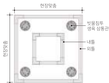
내부 평면도
