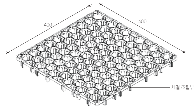
상세도면
