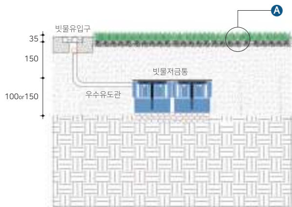
시공 단면도
