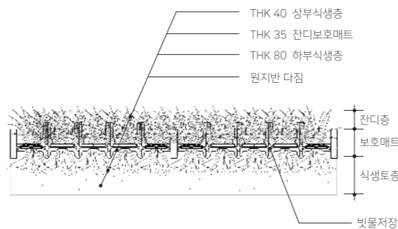
'A' 상세 단면도
