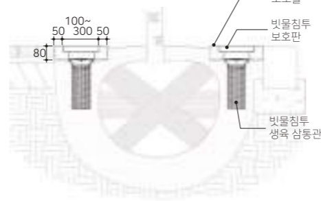
시공 단면도
